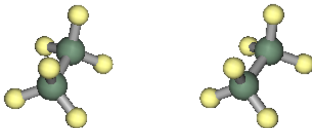
重なり型エタン(平行法)
